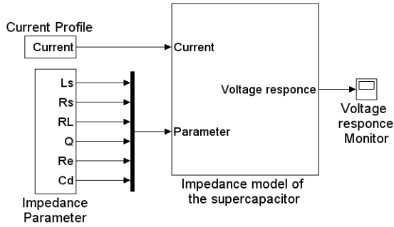
그림 11 Matlab/Simulink 구성도 Fig. 11 Matlab/Simulink Block diagram
