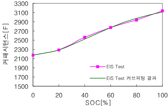
그림 8 Maxwell 슈퍼커패시터(2.7V 2600F)의 충전상태별 정전용량(0.01Hz, 20°C)
