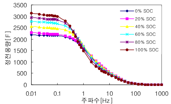
그림 7 Maxwell 슈퍼커패시터(2.7V 2600F)의 주파수 및 전압별 정전용량(20°C)
