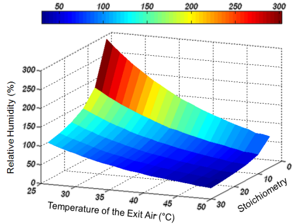
그림 5 화학량론과 출구 공기 온도에 따른 상대습도 그래프 Fig. 5 A graph of relative humidity versus temperature and stoichiometry
